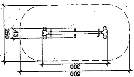
HUSTAWKA WAŻKA
