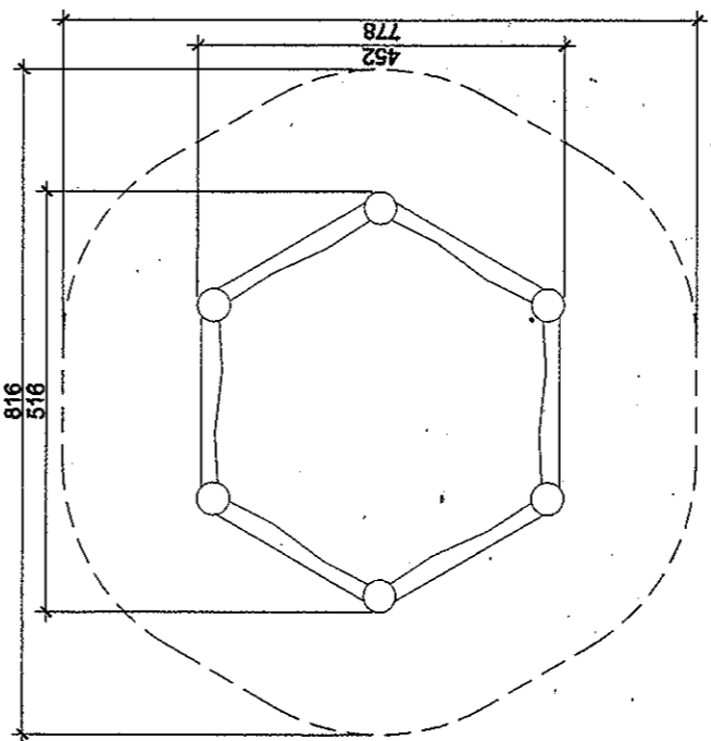
PIASKOWNICA SZEŚCIOKĄTA
