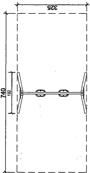
HUSTAWKA PODWÓJNA
