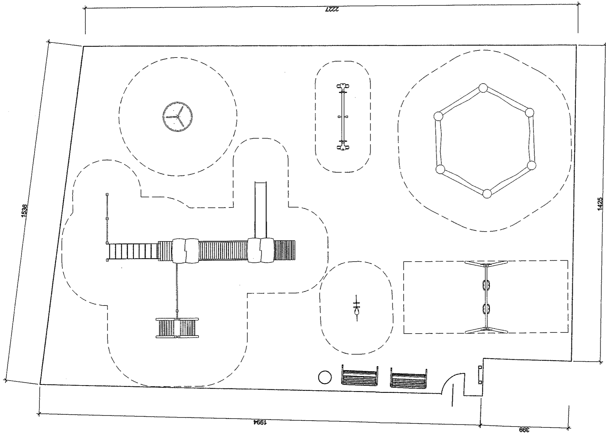
RZUT PRZEZIEMIA WRAZ Z STREFAMI BEZPIECZEŃSTWA
