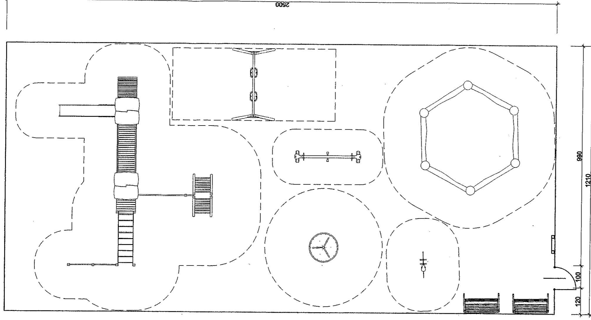
RZUT PRZEZIEMIA WRAZ Z STREFAMI BEZPIECZEŃSTWA
